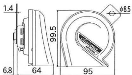
寸法図
