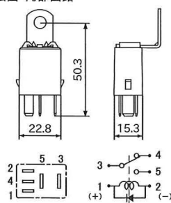
寸法図・内部回路
