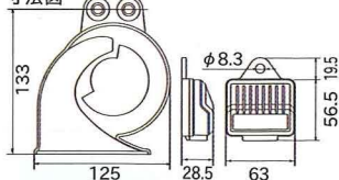
寸法図
