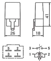
寸法図・内部回路
