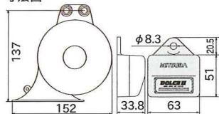
寸法図
