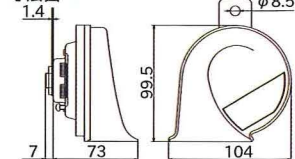
寸法図
