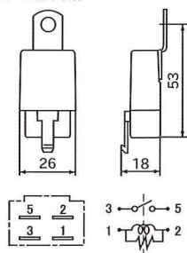
寸法図・内部回路
