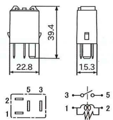
寸法図・内部回路
