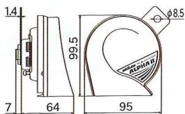
寸法図
