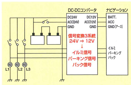
DDS-212A 入出力ケーブル 付属品
