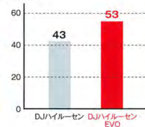
■ 試験滴下時の浸透度合い比較 高さ(mm)
