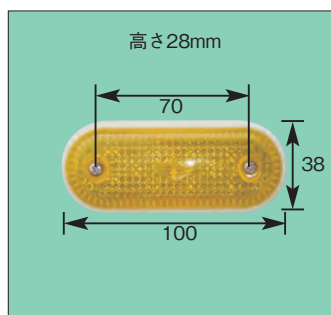
P-8023 (24V) 黄 LED 3個
